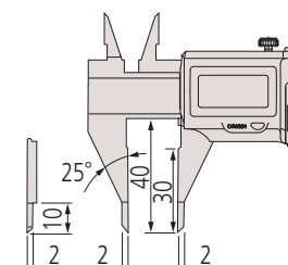
Špičaté měřicí čelisti
