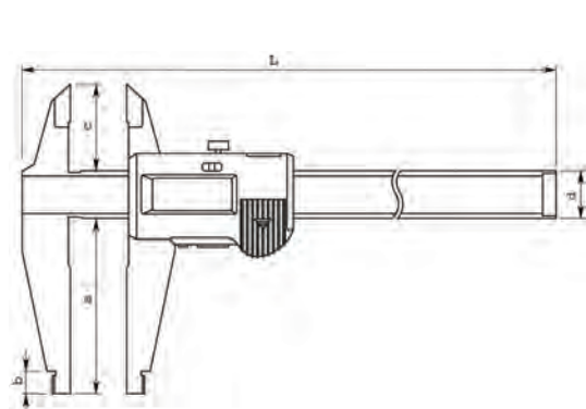
Zaoblené měřicí plochy na měření vnitřních rozměrů
