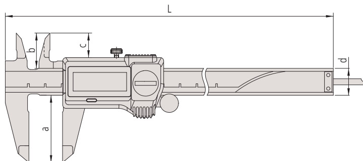
Měřicí čelisti osazené tvrdokovem
