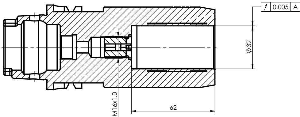
SCHNITT A-A
